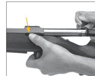
Нажмите на переднюю часть стоппера затвора для вставки или снятия затвора.
