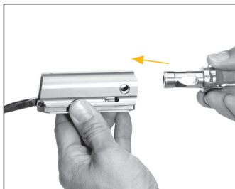
Inserire l'otturatore come illustrato
