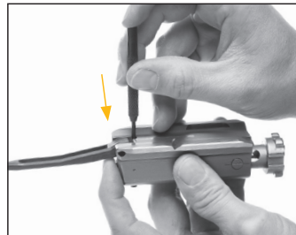
Tryck ut låsstiftet.
