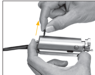
Dra ut slagstiftets låsstift.
