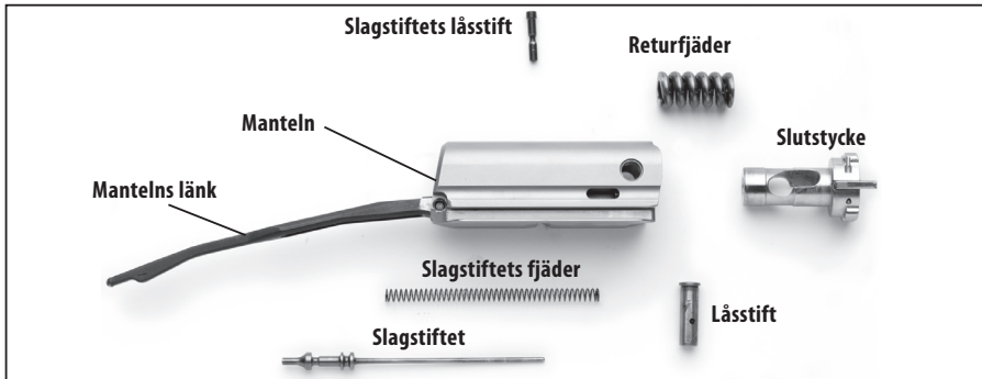
Manteln visas demonterad för rengöring.
